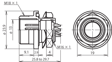
NJW-16 ■ -RBM
