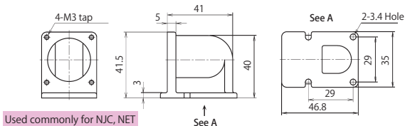
NJC-28-L za
