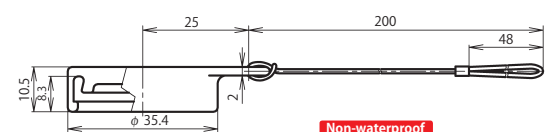
Adapter rubber cap : NRW-28-AdCa
