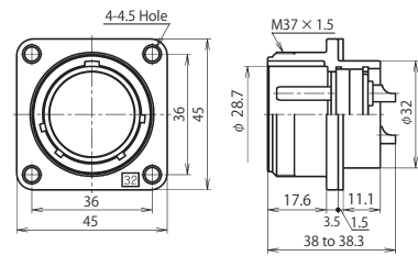
NJW-32 ■ -RM
