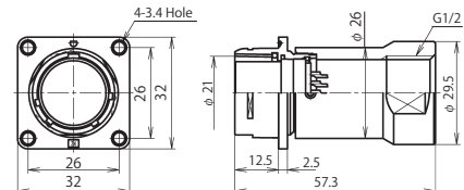
NR-24 ■ -GAd(F)F1/2 ( Note )
