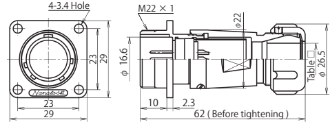
NJW-20 ■ -Ad(F)M □
