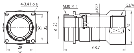
NJW-28 ■ -GAd(F)F3/4 ( Note )
