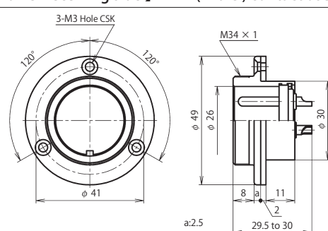
NWPC-30 ■ -R
