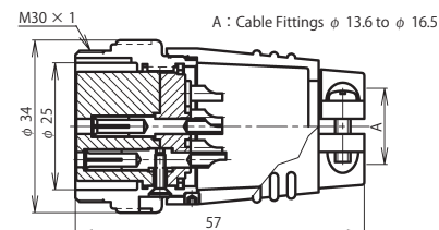
NET-28 ■ -AdF
