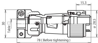
NAW-20 ■ -PFK □
