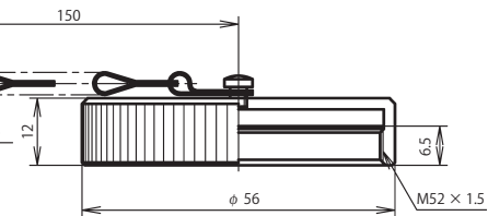
Receptacle cap : NWPC-44-RCa
