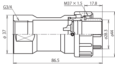
NJW-32 ■ -GPF3/4 ( Note )
