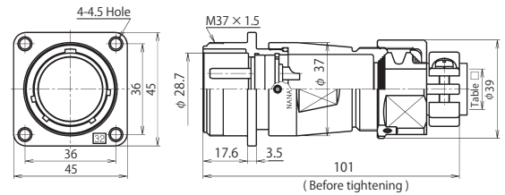
NJW-32 ■ -Ad(F)M □
