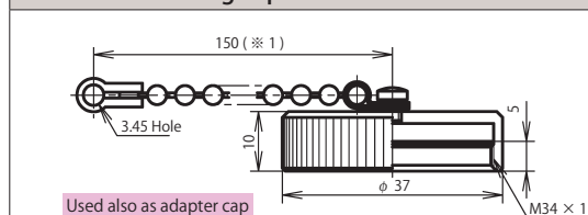
Plug cap : NWPC-30-PCa
