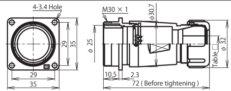
NJW-28 ■ -Ad(F)FK □
