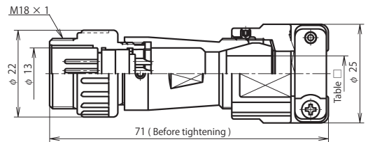
NJW-16 ■ -AdMK □
