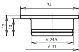
Plug cap : NR-24-PCa • 1
