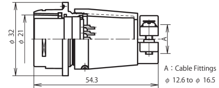
NR-24 ■ -AdF
