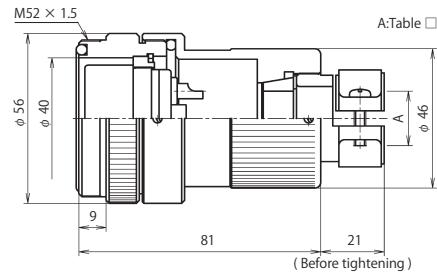
NWPC-44 ■ -AdF □
