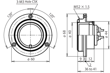
NWPC-44 ■ -RF
