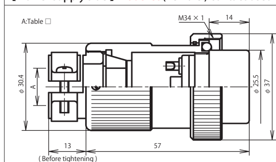
NWPC-30 ■ -P □
