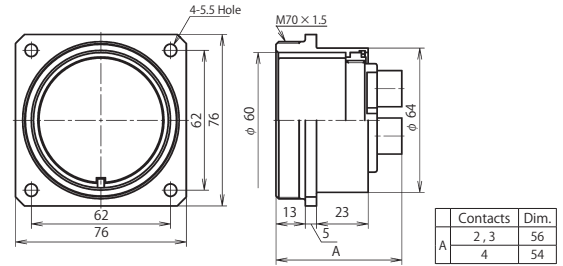
NCS-64 ■ -RF
