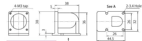
NJC-24-L za
