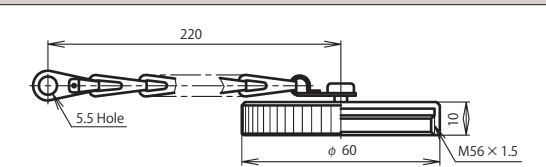
Receptacle cap : NT-50-RCa
