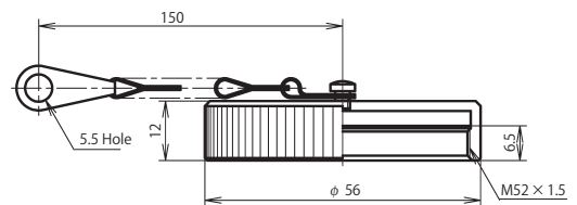
Adapter cap : NWPC-44-AdCa
