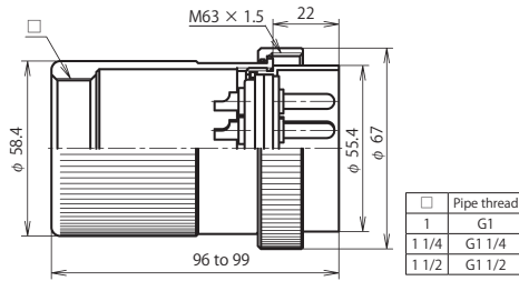
NCS-60 ■ -GPM □ ( Note )
