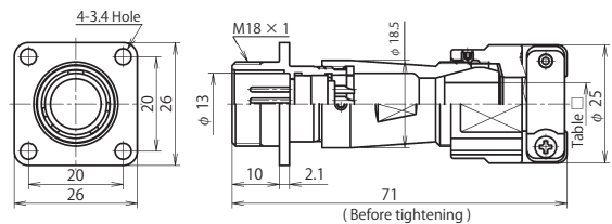
NJW-16 ■ -Ad(F)MK □
