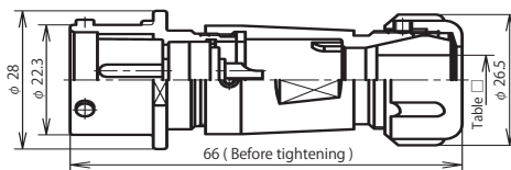
NAW-20 ■ -AdM □
