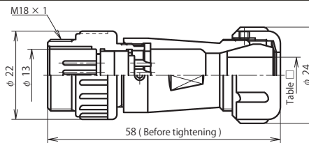
NJW-16 ■ -AdM □
