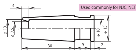
Cable bushing : NJC-20-CB
