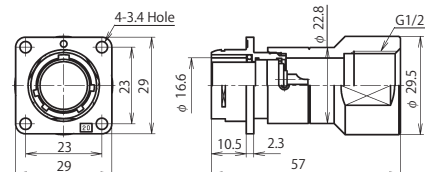
NR-20 ■ -GAd(F)F1/2 ( Note )
