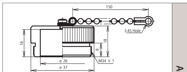
Plug cap : NWPC-30-PCa
